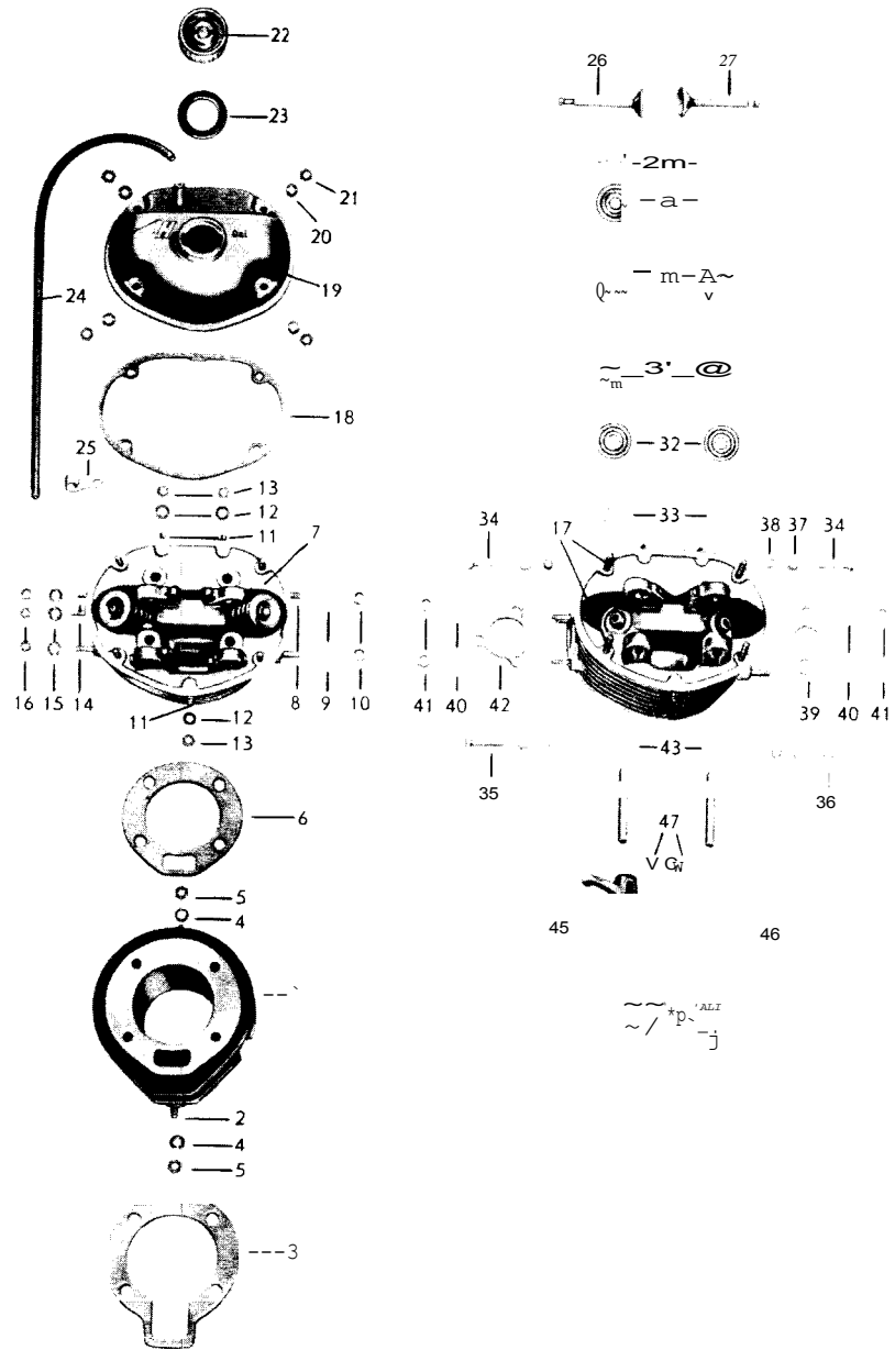
Tafel 3 Zylinderkopf / Zylinderkopf
